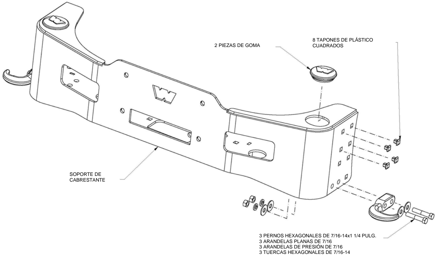
Figura A: Vista expandida del modelo de bastidor grande
