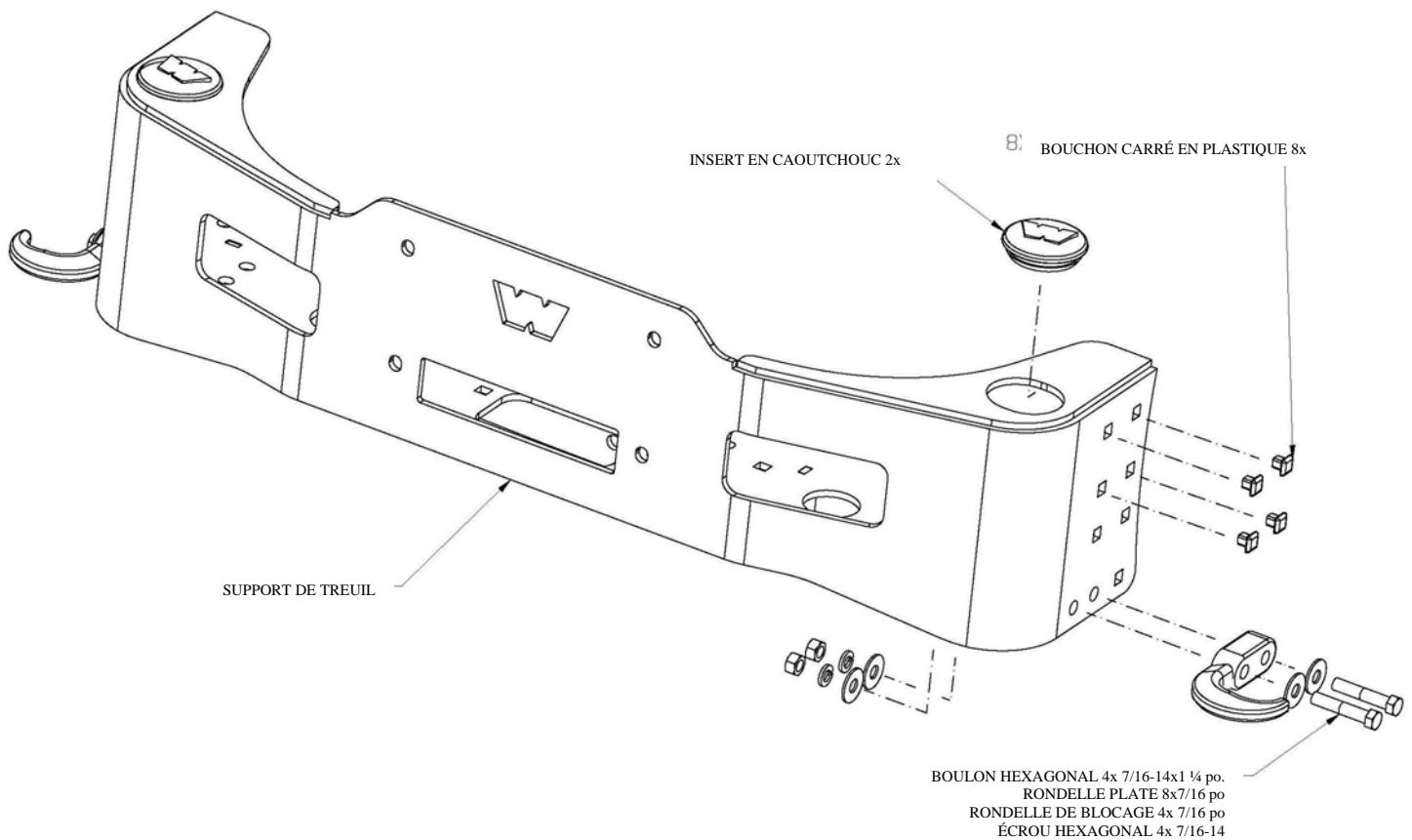
Figure A : Vue éclatée châssis large
